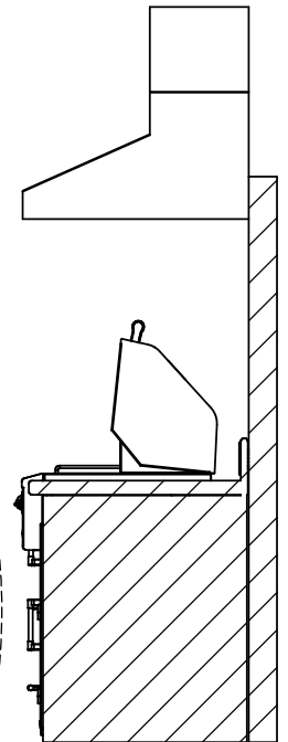
SECTION D-D
