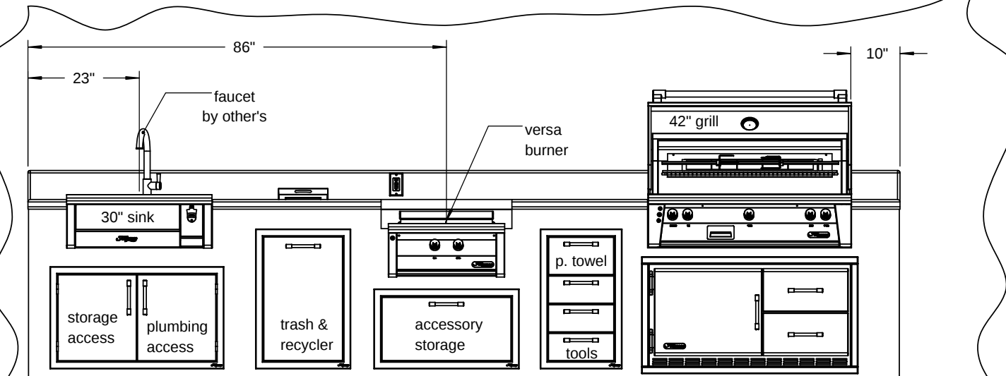
SECTION A-A
